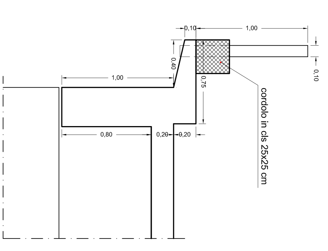
Particolare sbalzo carreggiata e guard rail Scala 1:20
